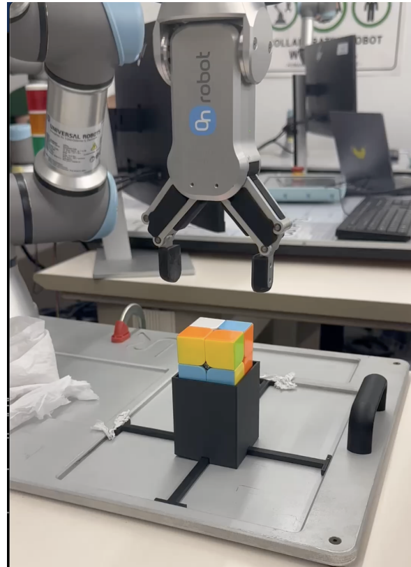
(b) Execució amb el robot real UR3
