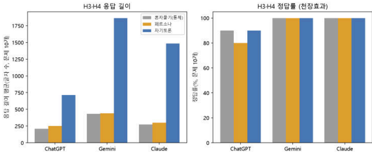
그림 6. H3·H4 응답 길이와 정답률
