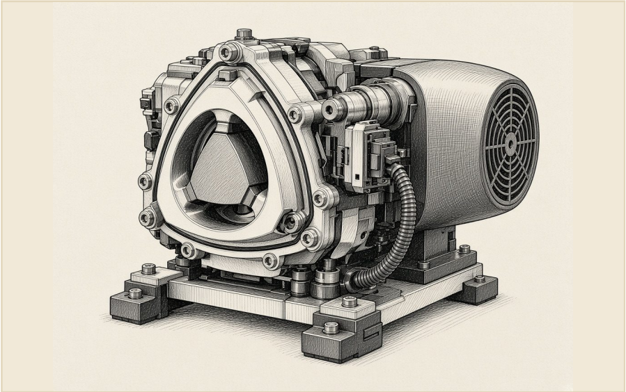
마쓰다 8C 로터리 발전기. 주인공에서 조연으로 살아남는 엔진.
