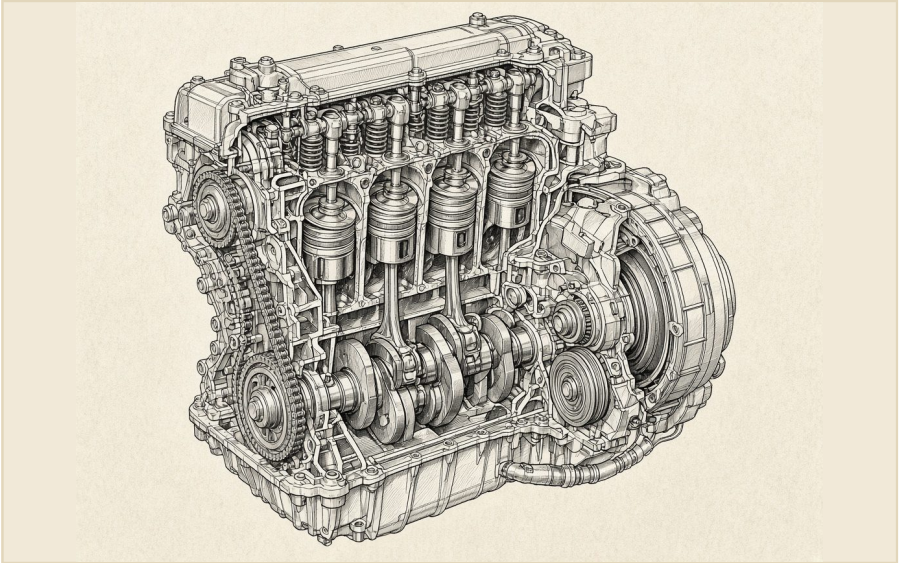
토요타 A25A-FXS. 효율의 시대를 상징하는 엔진.
