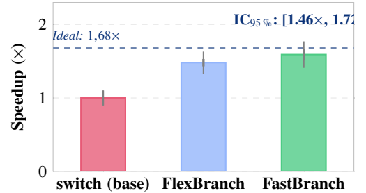
Figura 4. Speedup relativo al switch nativo con IC Bootstrap al 95%. Cohen’s d = 1,07 indica diferencia grande. La línea punteada muestra el límite sin dispatch condicional. IC empírico para FastBranch : [1,46\times, 1,72\times] .
