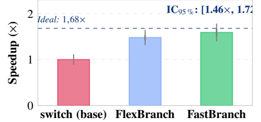
Figura 4. Speedup relativo al switch nativo con IC Bootstrap al 95 %. Cohen's d = 1,07 indica diferencia grande. La línea punteada muestra el límite sin dispatch condicional. IC empírico para FastBranch : [1,46×, 1,72×].
