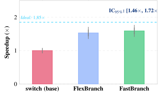
Figura 4. Speedup relativo al switch nativo con IC Bootstrap al 95%. Cohen's d = 1,07 indica diferencia grande. La línea punteada muestra el límite sin dispatch condicional. IC empírico para FastBranch : [1,46 \times , 1,72 \times ].
