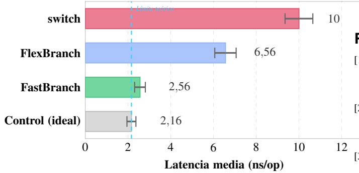
Figura 3. Latencia media por estrategia con intervalos de confianza empíricos al 95% (Bootstrap, B = 10000 ). La línea punteada indica el límite teórico (control directo sin dispatch ). FastBranch converge a este límite con diferencia estadísticamente significativa respecto al switch ( p < 0.0001 ). Se prescinde de la leyenda duplicada para mejorar la claridad visual.
