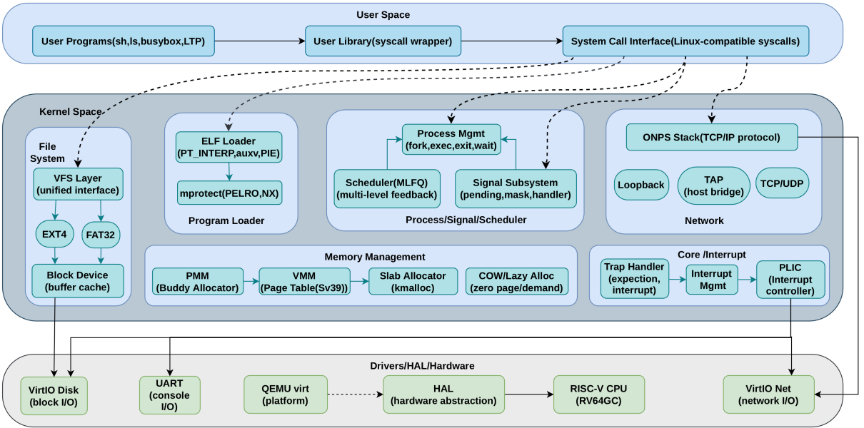
图 1.2: RuOS 决赛架构图
