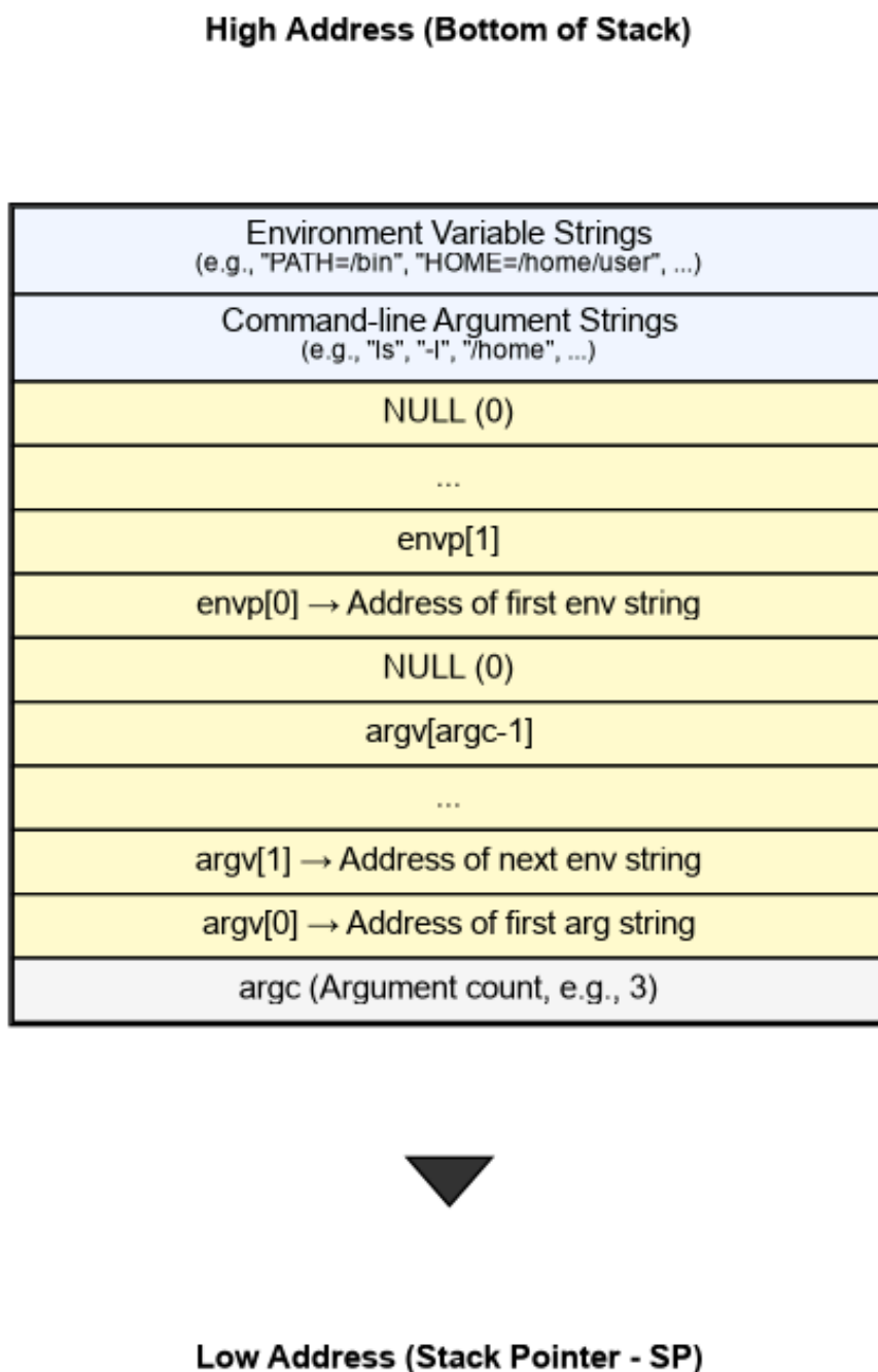
图 7.1: RuOS 用户栈布局图
