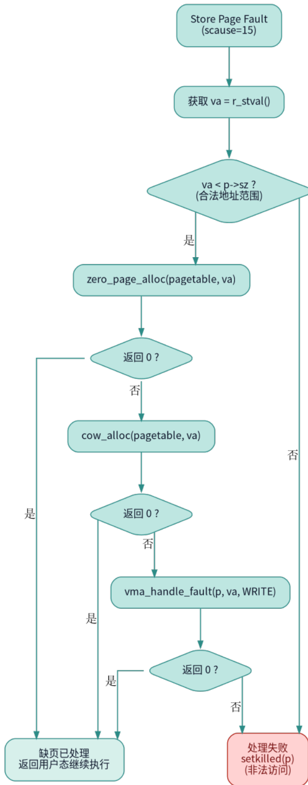
图 3.6: 缺页处理流程
