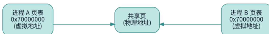
图 5.2: 共享内存映射图
