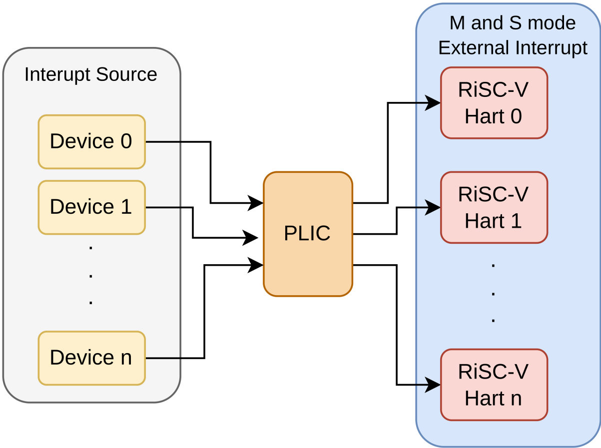
图 9.2: PLIC 中断工作机制
