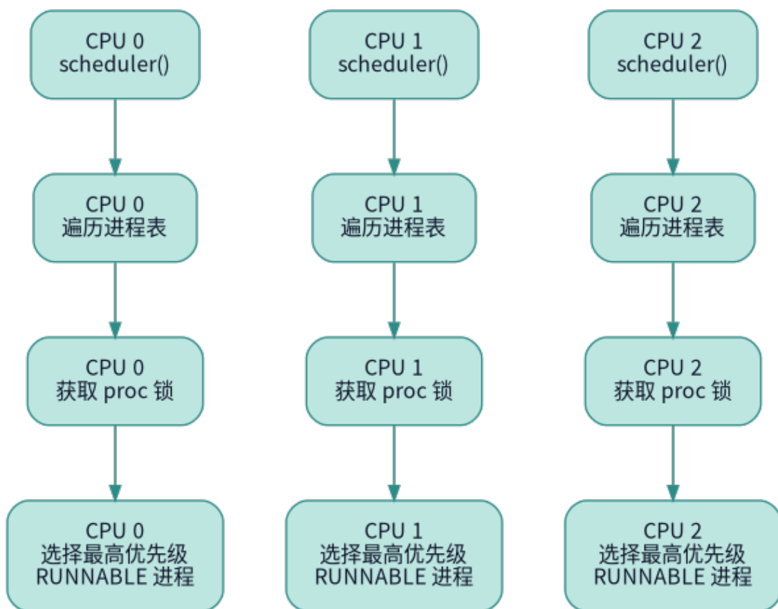
图 2.3: 多核调度示意图
