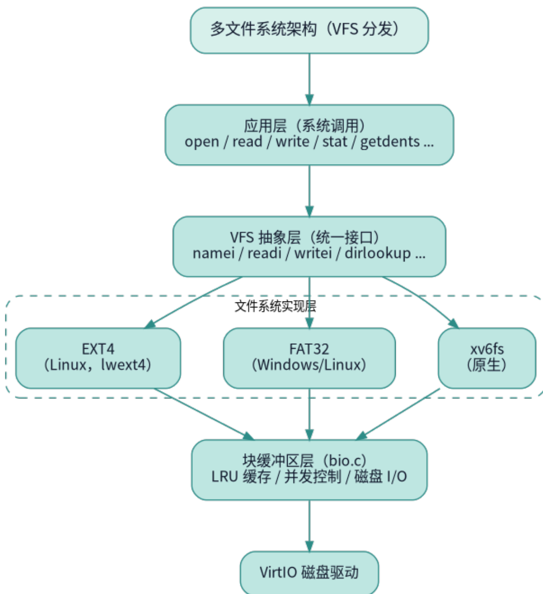
图 4.1: RuOS 的 VFS 设计
