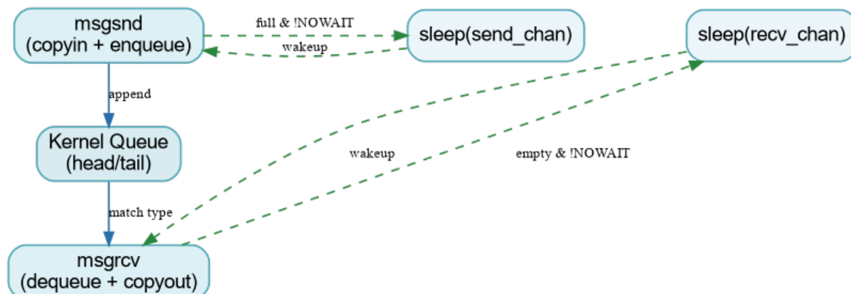
图 5.5: 消息队列收发与阻塞/唤醒流程图
