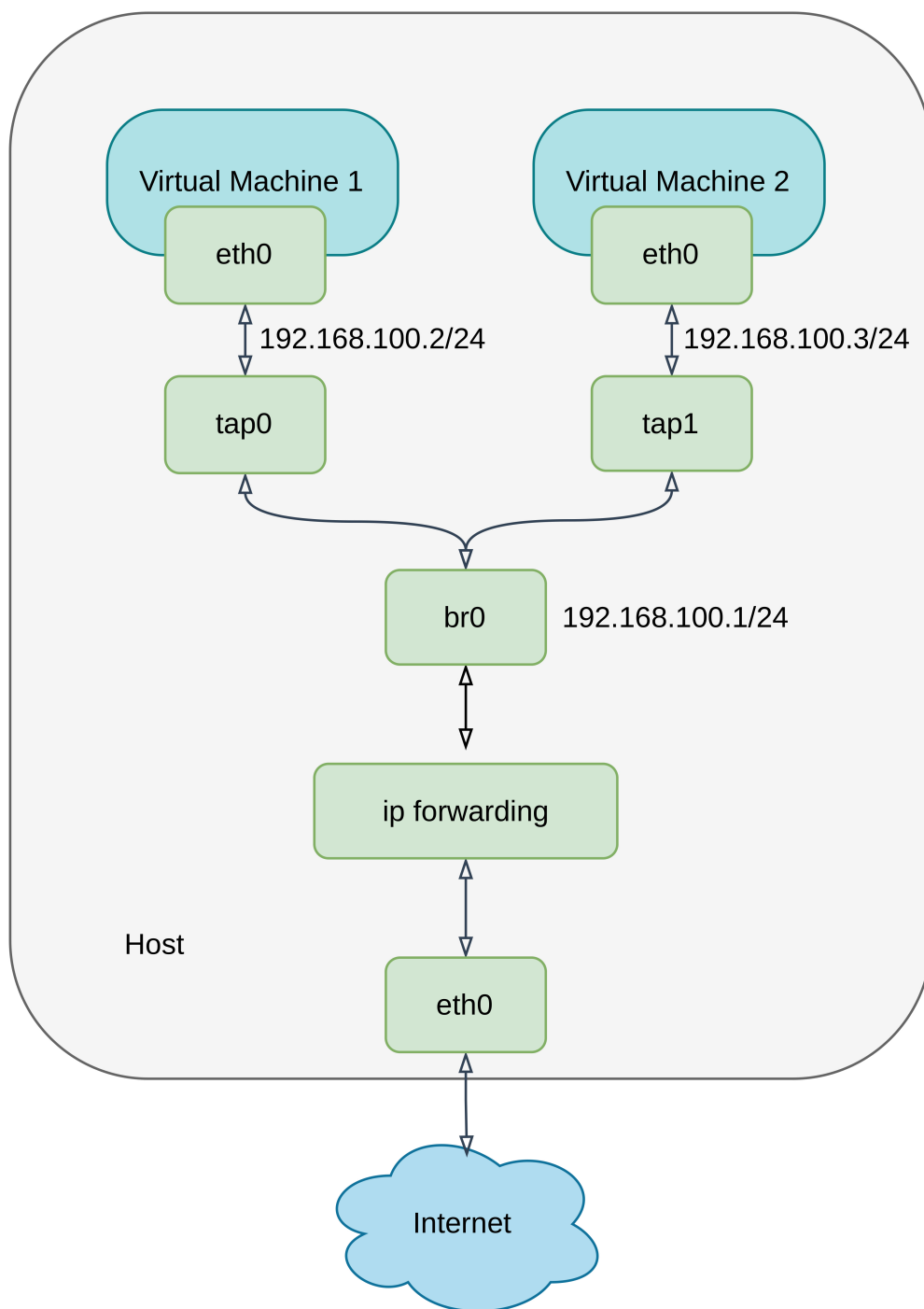
图 6.2: QEMU Tap Networking 拓扑图
