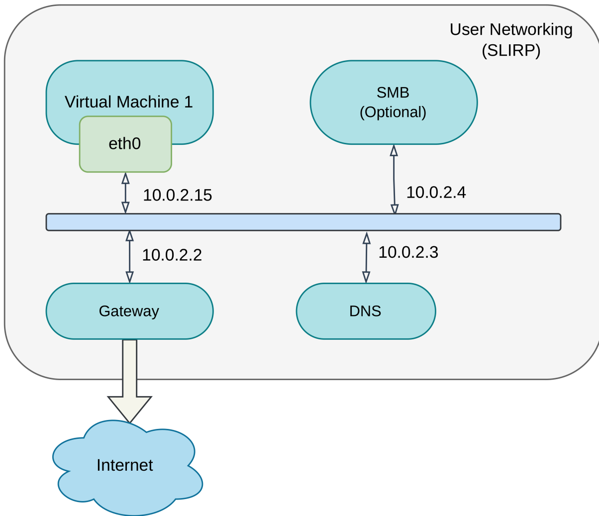
图 6.1: QEMU User Networking 拓扑图
