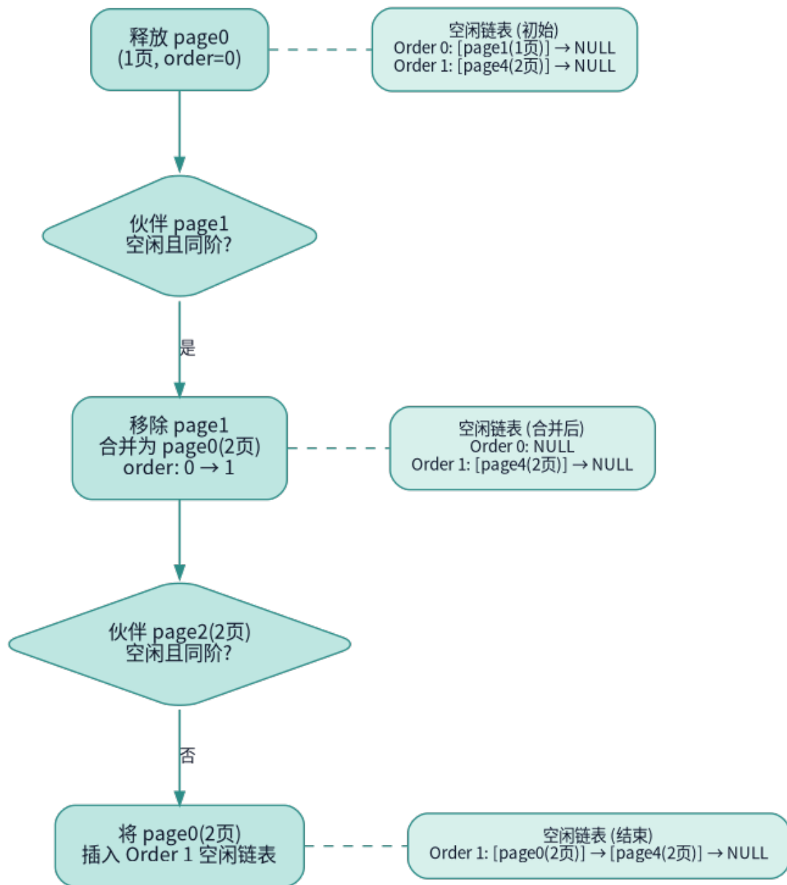
图 3.3: Buddy 合并过程
