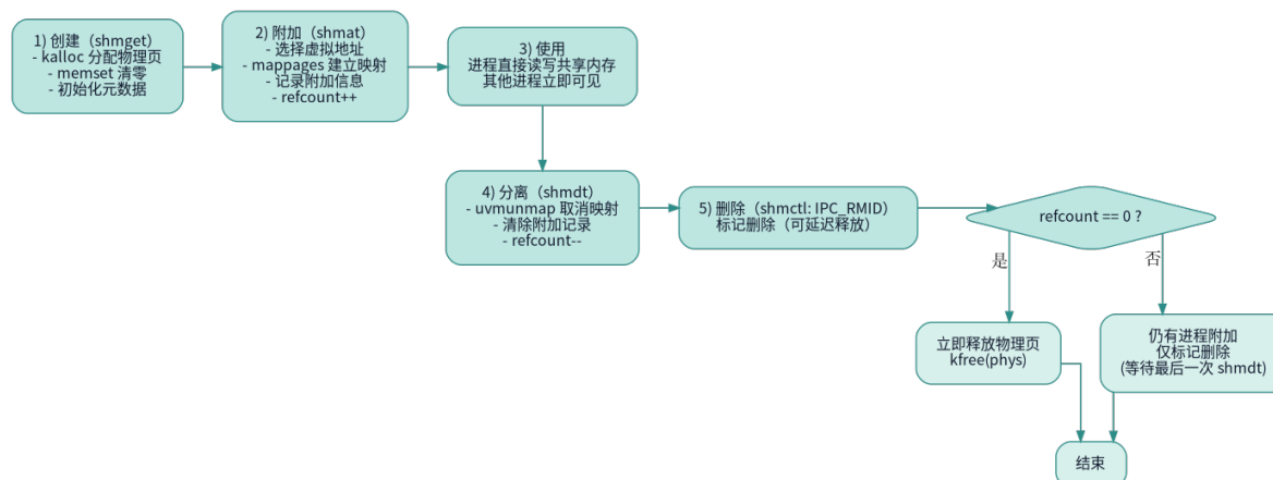
图 5.3: 共享内存生命周期
