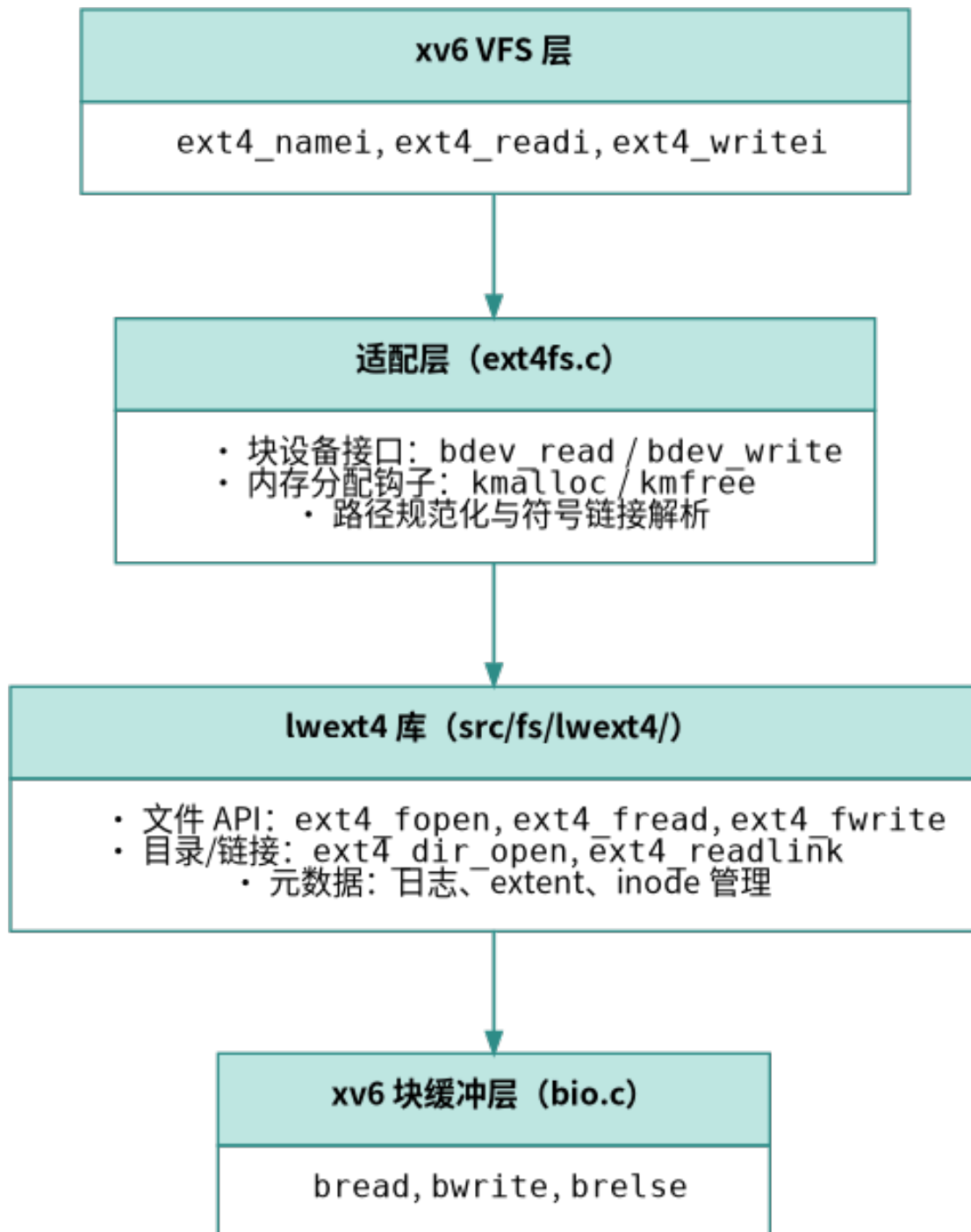
图 4.5: RuOS 适配 EXT4 fs
