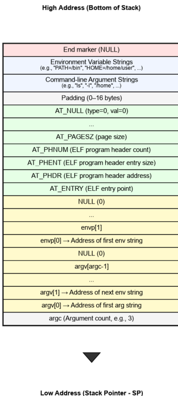
图 7.1: RuOS 用户栈布局图
