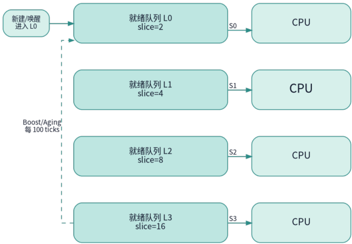
图 2.2: MLFQ 多级反馈队列（实现要点）
