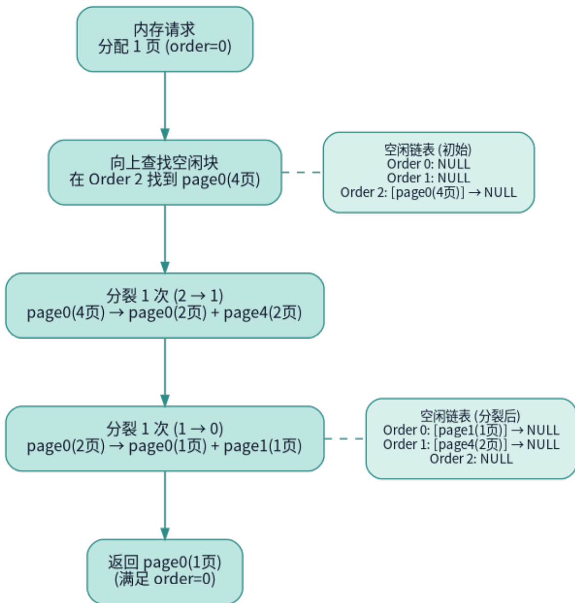
图 3.2: Buddy 分配过程
