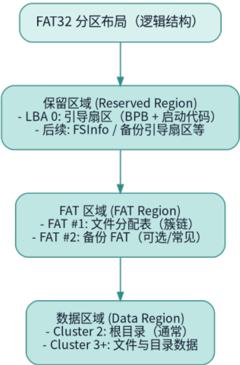
图 4.2: FAT32 分区布局
