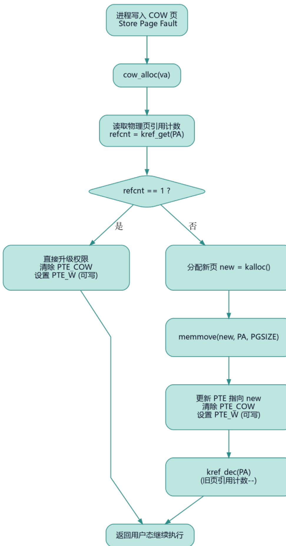
图 3.5: COW 处理流程图
