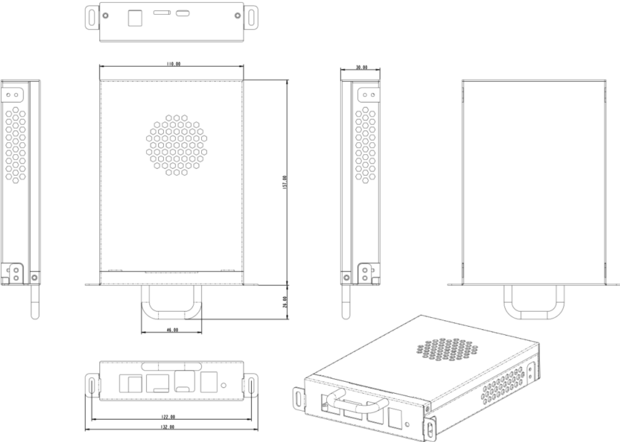
图 2: 产品六视图
