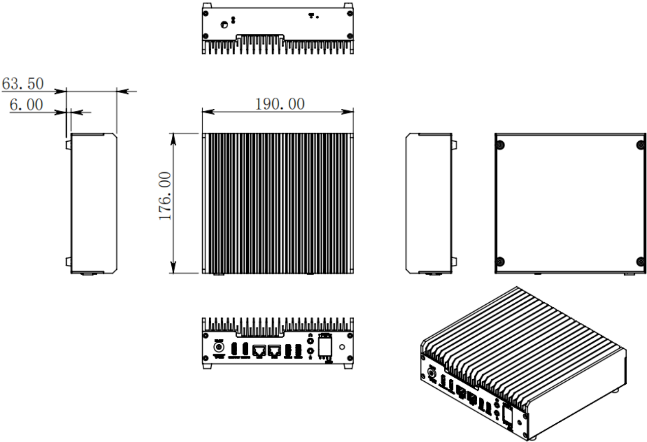
图 2: 产品六视图
