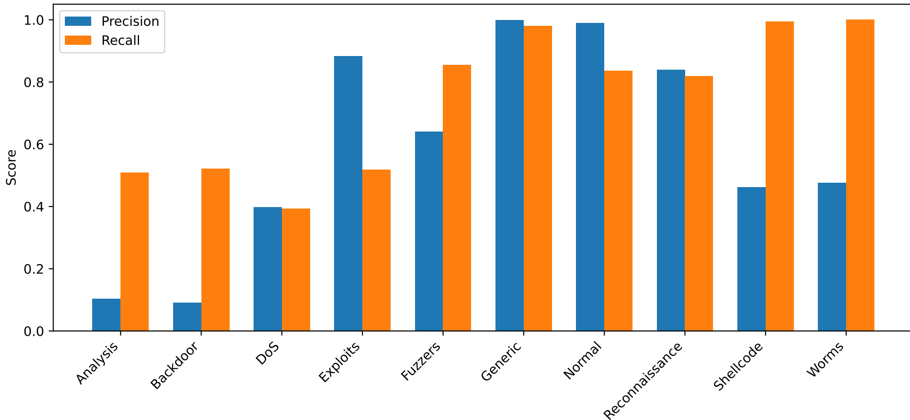
Precision & Recall per class
