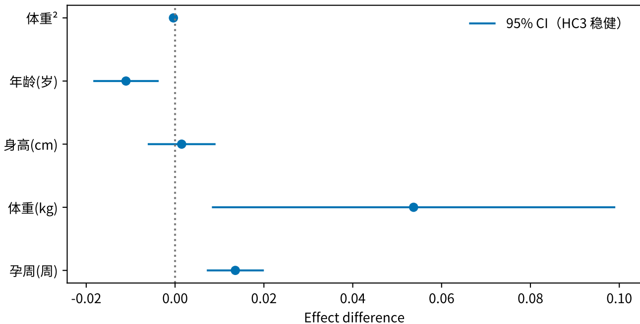
扩展模型 (E4_wh_quad) ln(Y浓度) 回归系数及 95% CI
