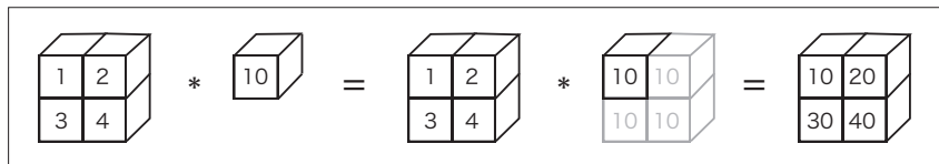
图 1-1 广播的例子: 标量 10 被当作 2 \times 2 的矩阵
