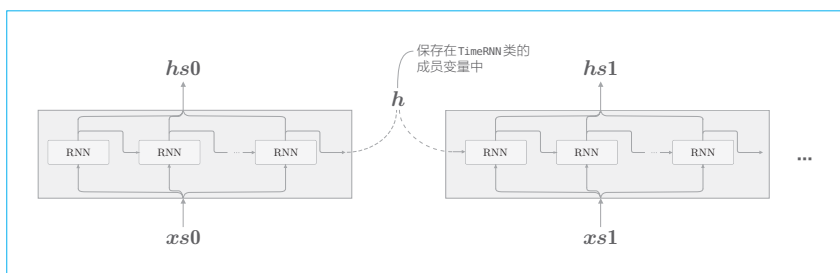
图 5-22 Time RNN 层将隐藏状态 h 保存在成员变量中，以在块之间继承隐藏状态
