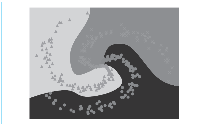
图1-33 学习后的神经网络的决策边界（用不同颜色描绘神经网络识别的各个类别的区域）
