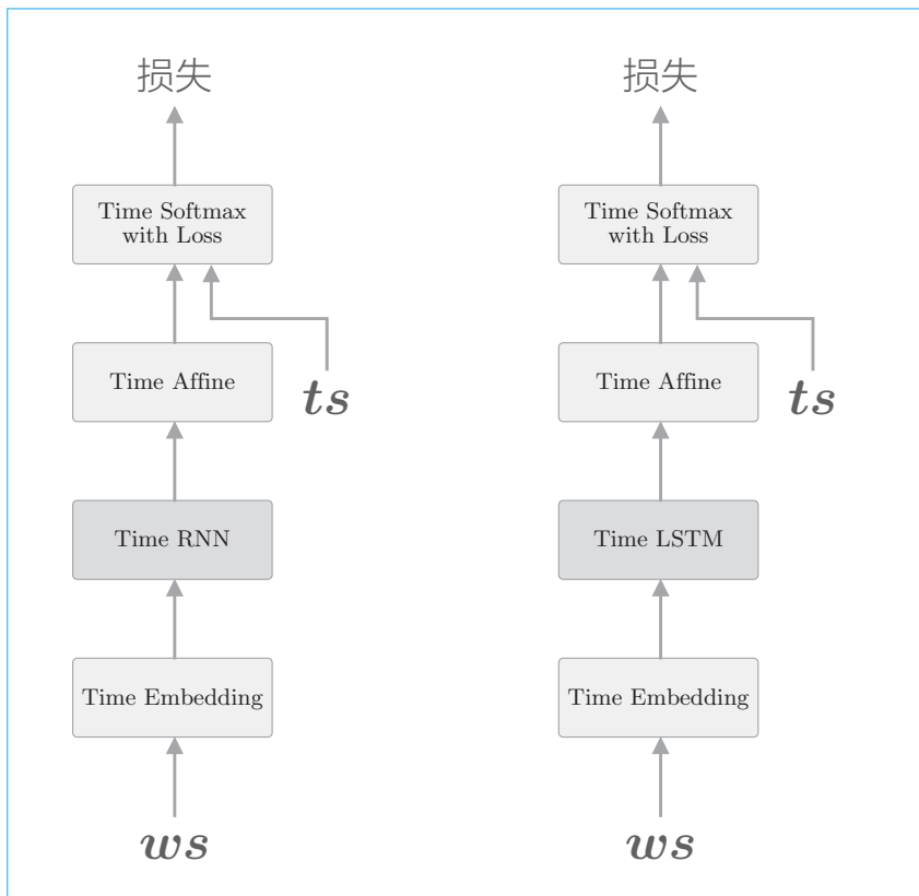
图 6-26 语言模型的网络结构。左图是上一章创建的使用 Time RNN 的模型，右图是本章创建的使用 Time LSTM 的模型
