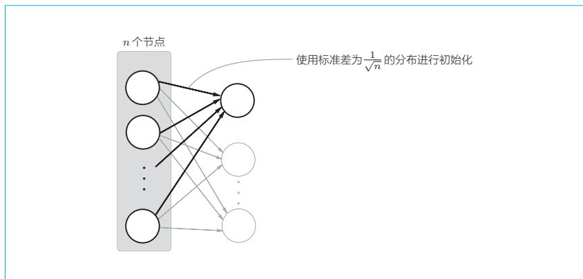
图 5-31 Xavier 初始值：在上一层有 n 个节点的情况下，使用标准差为 \frac{1}{\sqrt{n}} 的分布作为初始值
