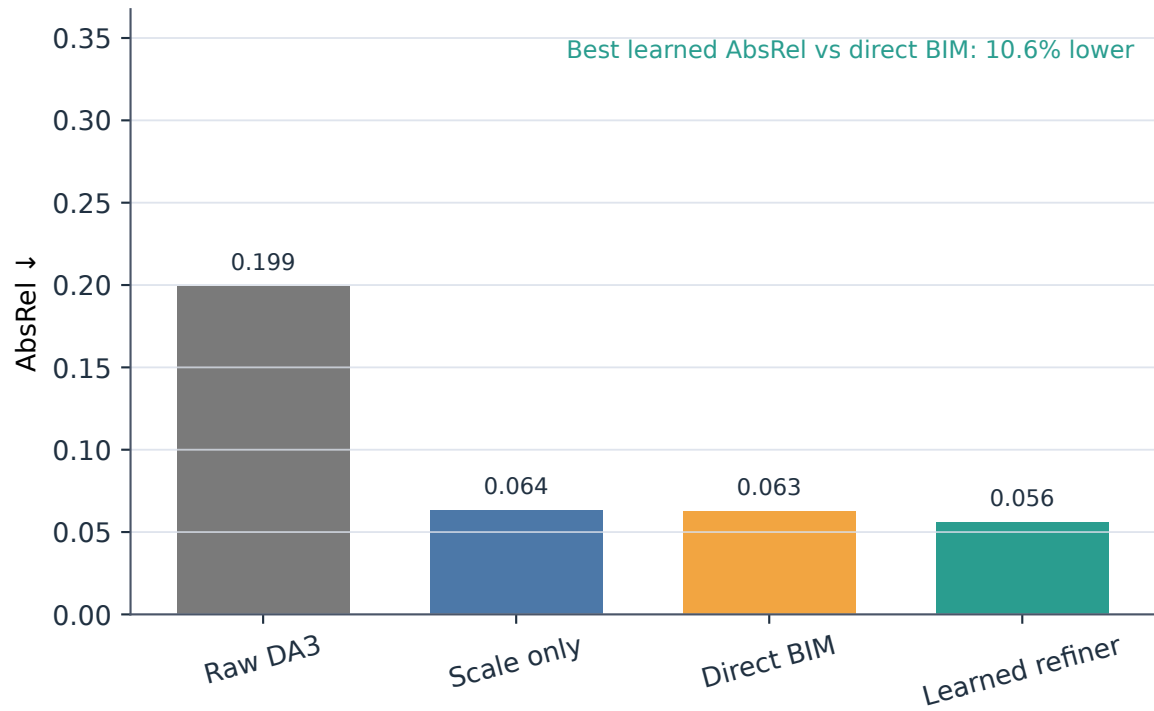
SLABIM
