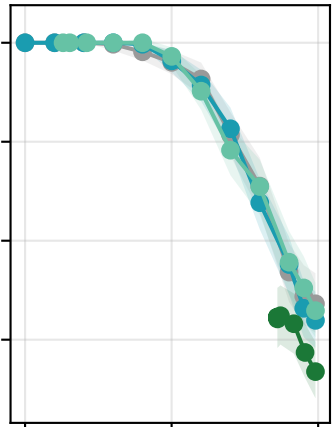
GPQA-Diamond
