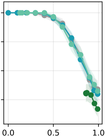
GPQA-Diamond
