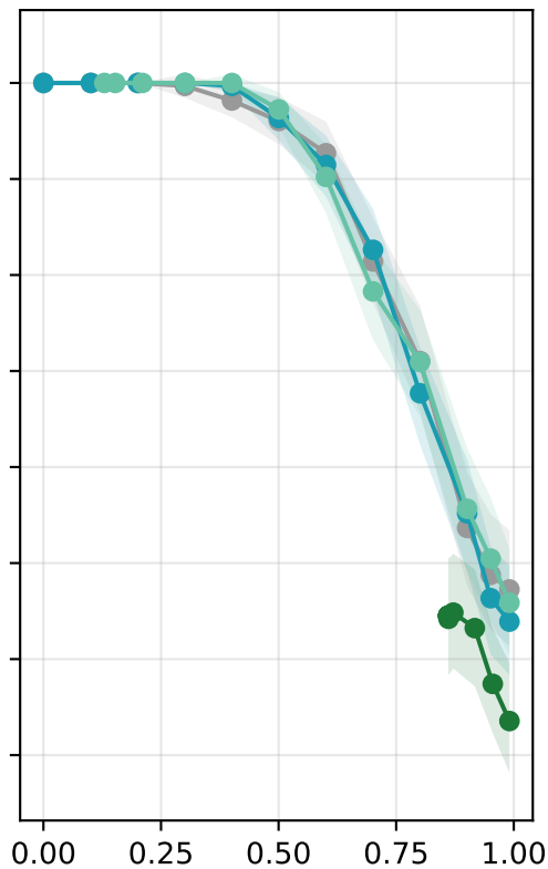
GPQA-Diamond
