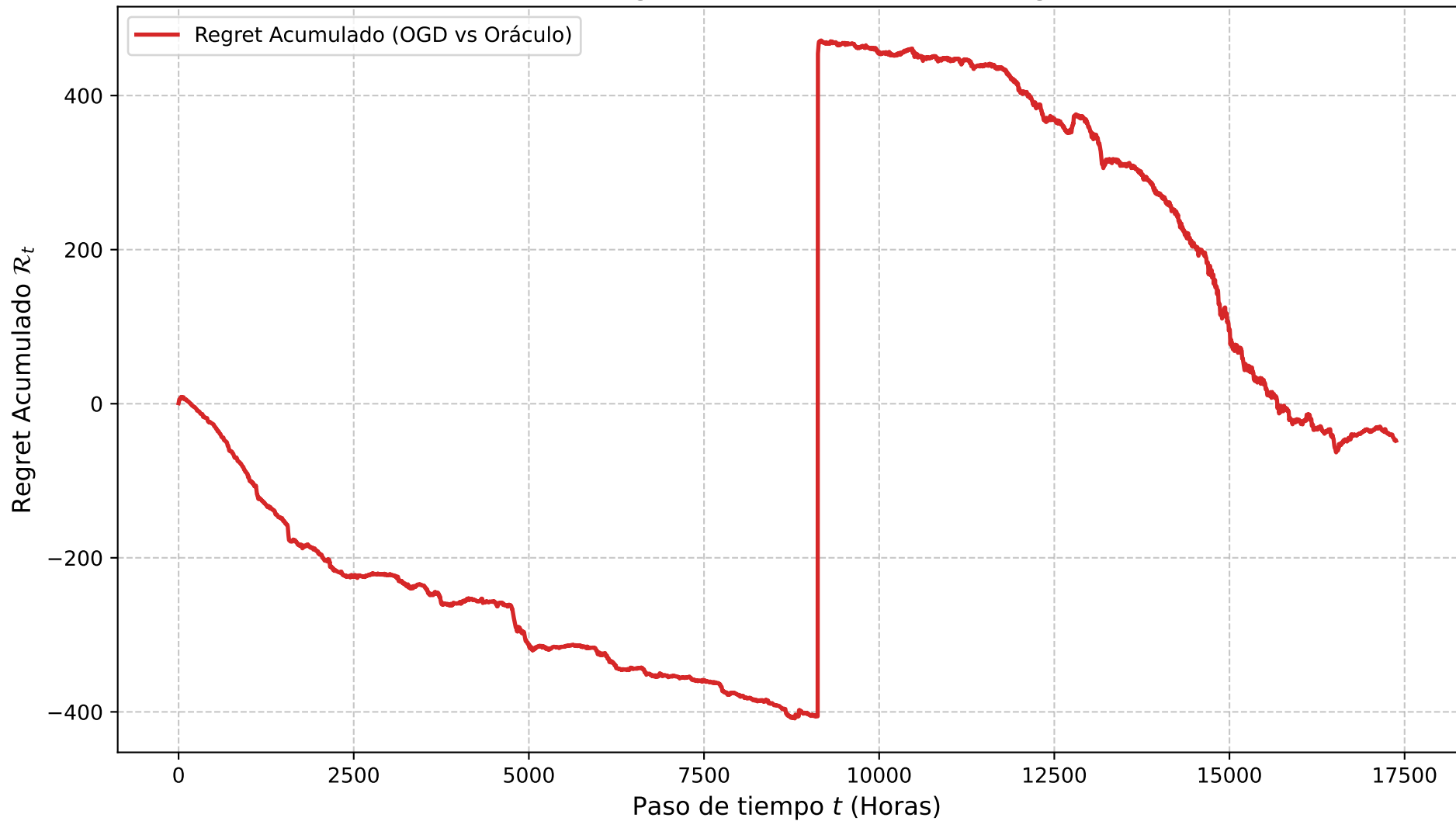
Evolución del Regret de OGD en Bike Sharing Demand
