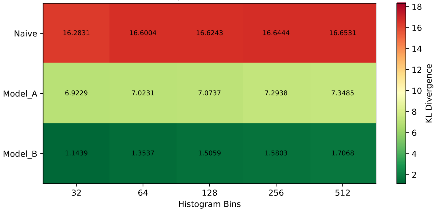
KL Divergence (Bins x Models)
