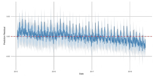
(d) Residuals over time
