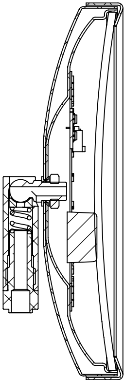
SEÇÃO A-A
