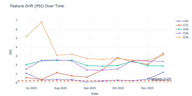
Fig. 6: Evolució del PSI per a les 5 variables principals del model. Línia discontinua vermella: líndar de drift significatiu (PSI > 0.25).
