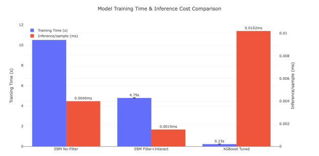
Fig. 5: Comparació de temps d'entrenament i latència d'inferència entre EBM (amb i sense filtratge) i XGBoost.
