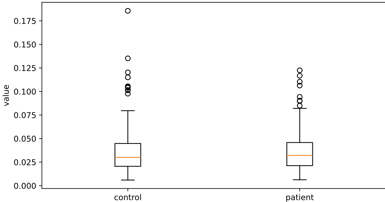
apq5_shimmer
