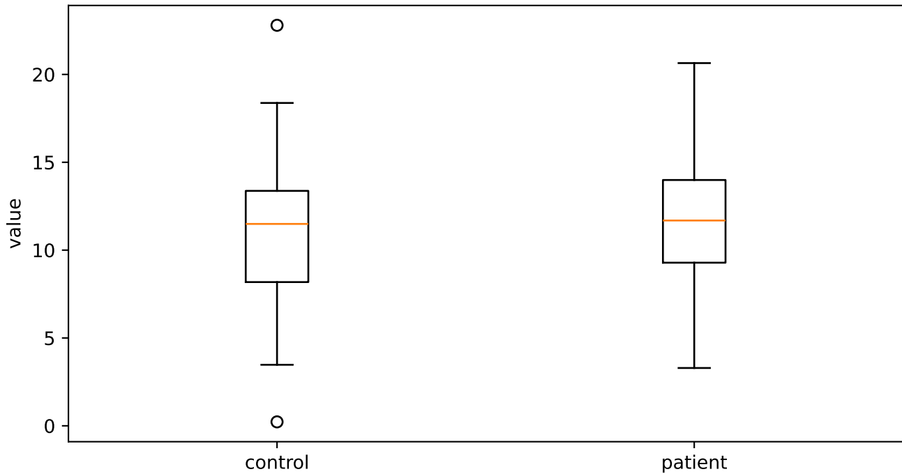
std_intensity_db
