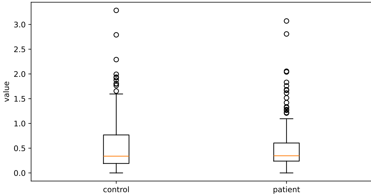
StddevUnvoicedSegmentLength
