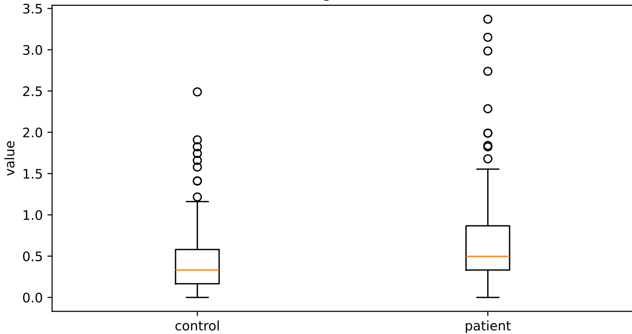
VoicedSegmentsPerSec
