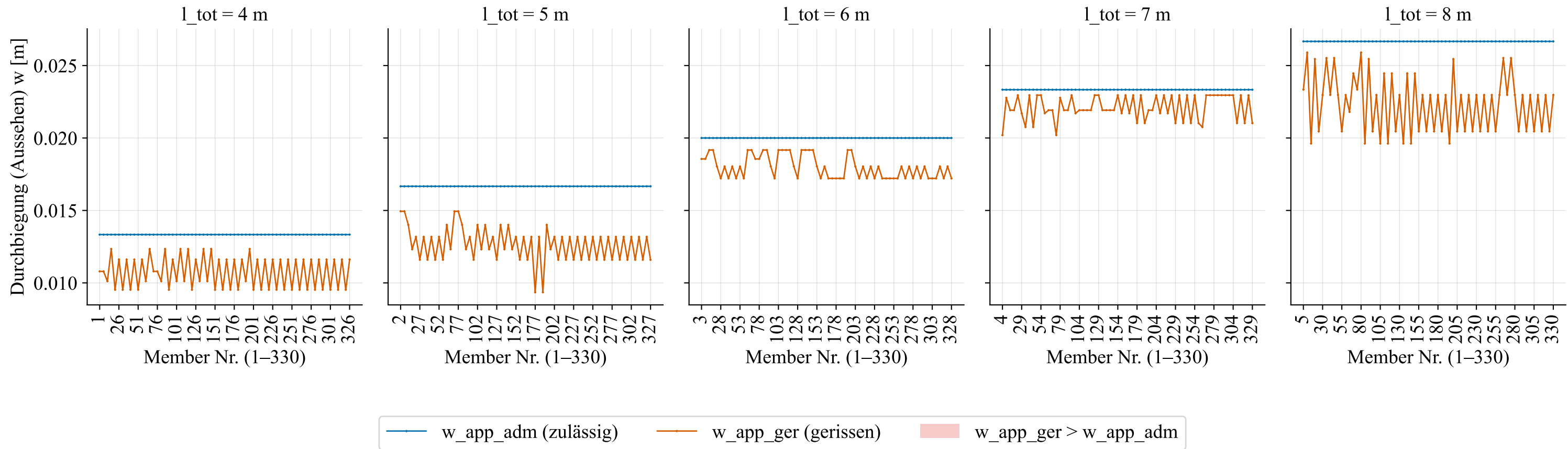
Durchbiegung w_app_adm (zulässig) vs. w_app_ger (gerissen) je Member, kategorisiert nach Spannweite (Members_rc_rec_simple_massiv)
