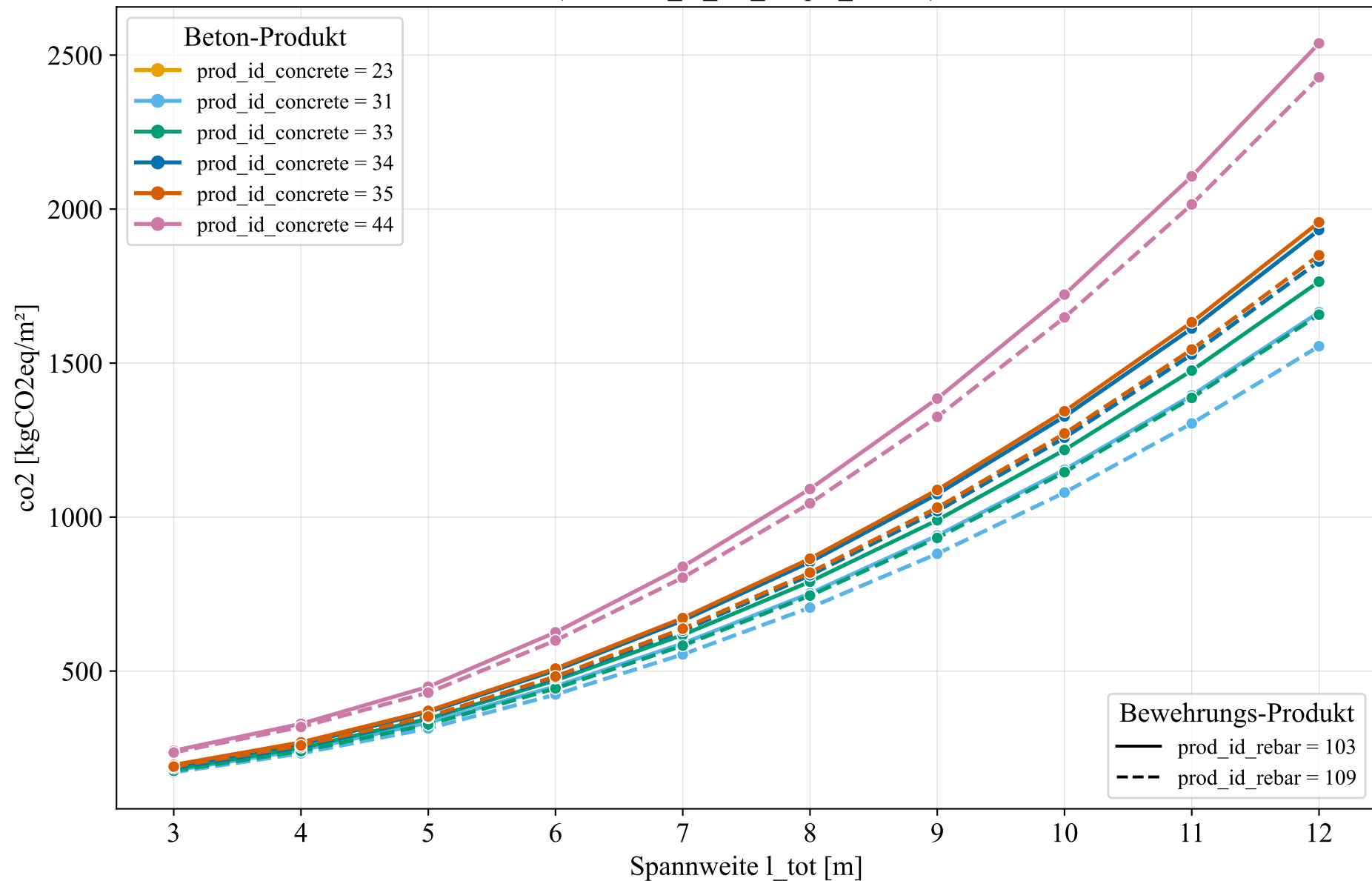
co2 vs. Spannweite, je Beton- und Bewehrungs-Produkt (Members_rc_rec_simple_massiv)
