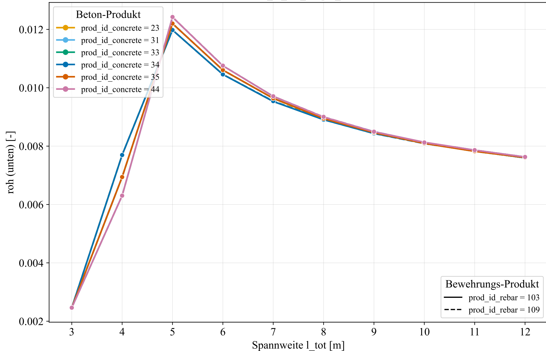
roh vs. Spannweite, je Beton- und Bewehrungs-Produkt (Members_rc_rec_simple_massiv)
