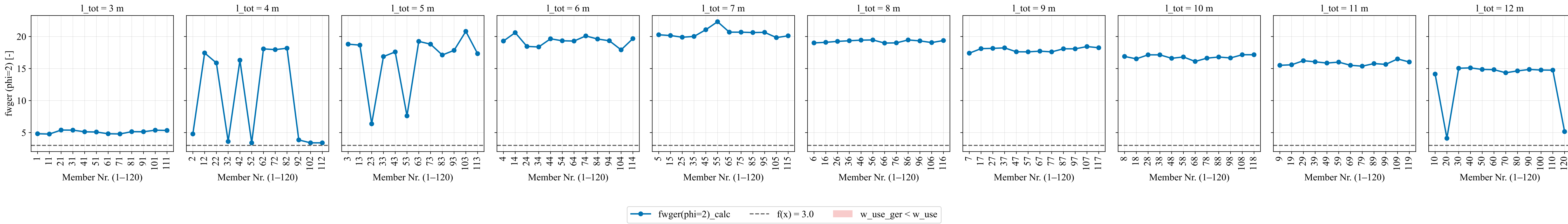
Faktor fwger(phi=2)_calc je Member, kategorisiert nach Spannweite (Members_rc_rib_simple_massiv)
