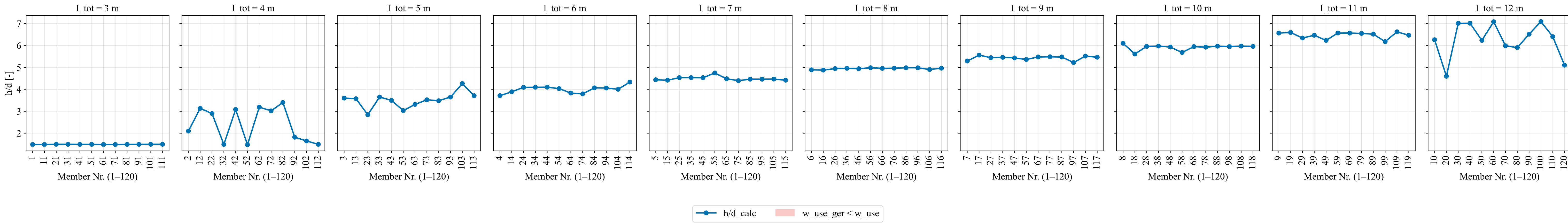
Verhaeltnis h/d_{\text{calc}} je Member, kategorisiert nach Spannweite (Members_rc_rib_simple_massiv)
