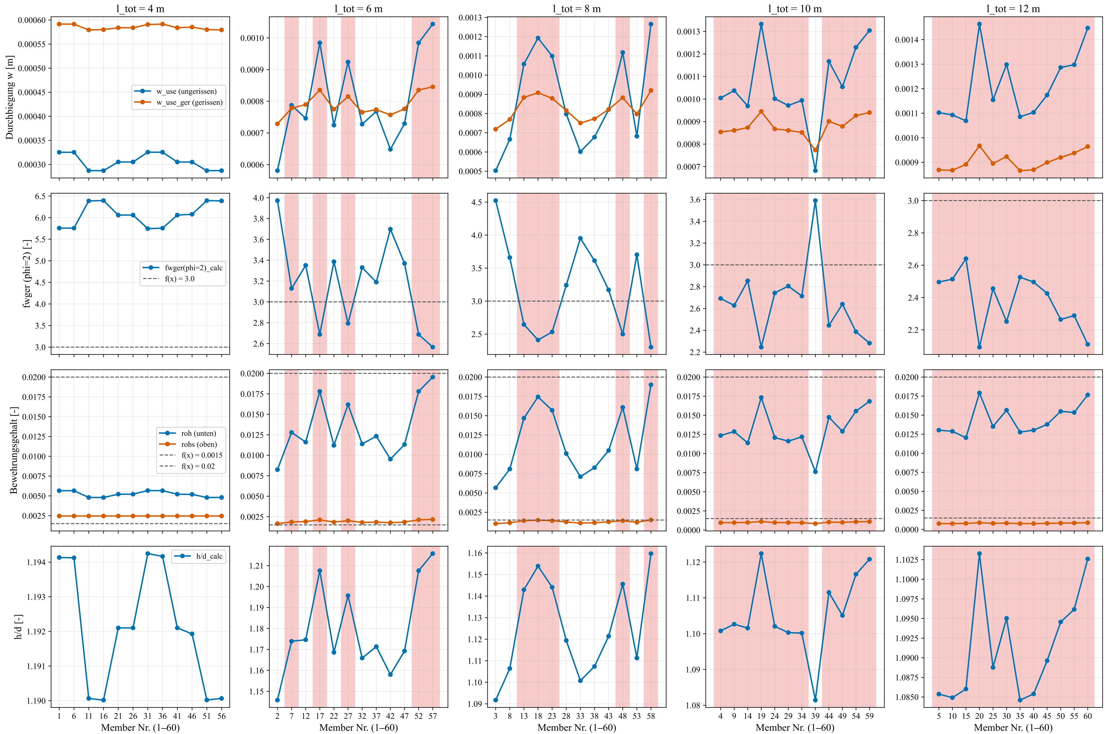
Übersicht: Durchbiegung, fwger(phi=2), Bewehrungsgehalt und h/d je Member, kategorisiert nach Spannweite
