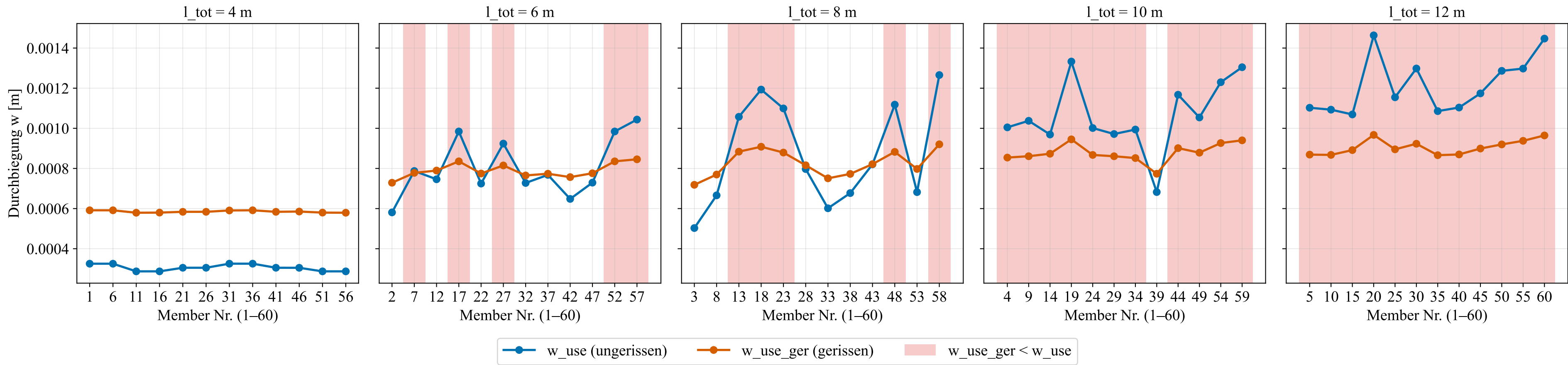
Durchbiegung w_{\text{use}} vs. w_{\text{use\_ger}} je Member, kategorisiert nach Spannweite
