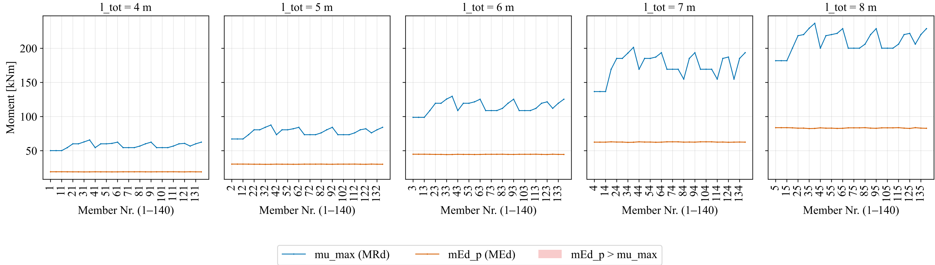
Biege widerstand \mu_{\max} (MRd) vs. Bemessungsmoment mEd_p (MEd) je Member, kategorisiert nach Spannweite (Members_wd_rec_simple_)
