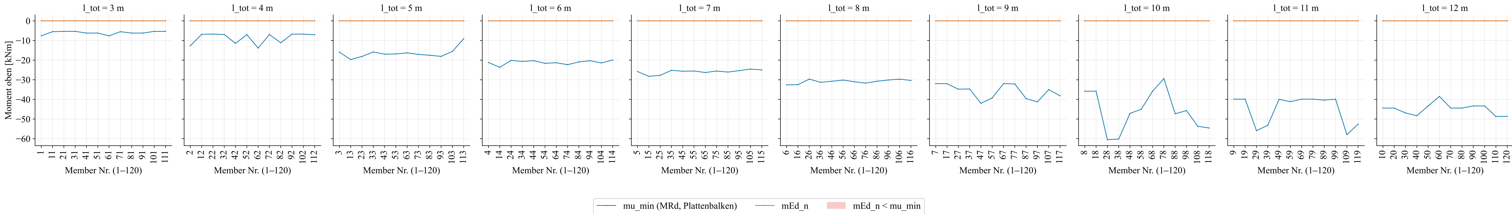
Biege widerstand \mu_{\min} (MRd, Plattenbalken) vs. Bemessungsmoment mEd_n je Member, kategorisiert nach Spannweite (Members_rc_rib_simple_massiv_bvar)
