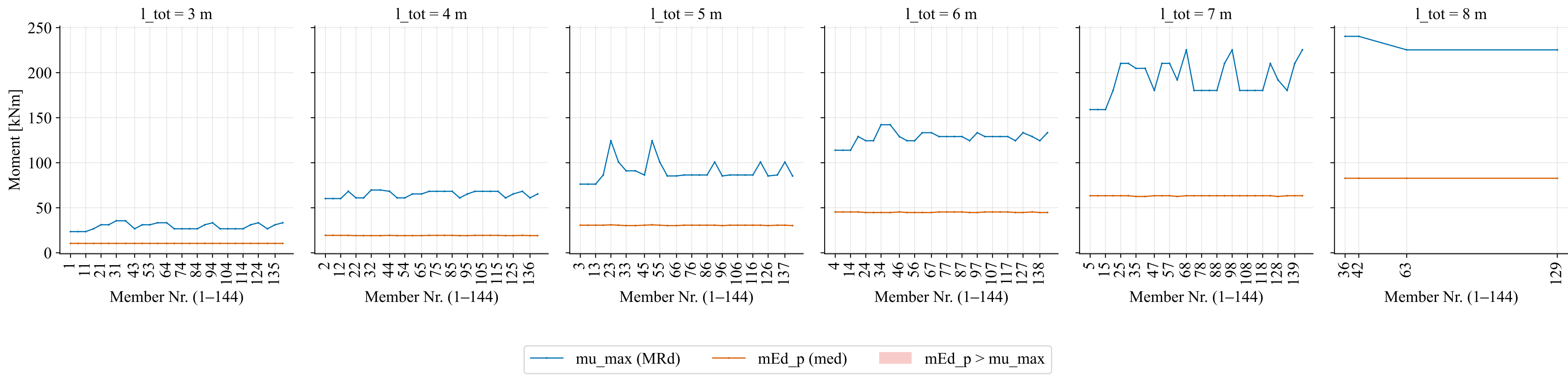
Biege widerstand \mu_{\max} (MRd) vs. Bemessungsmoment mEd_p (med) je Member, kategorisiert nach Spannweite (Members_wd_rec_simple_260902)
