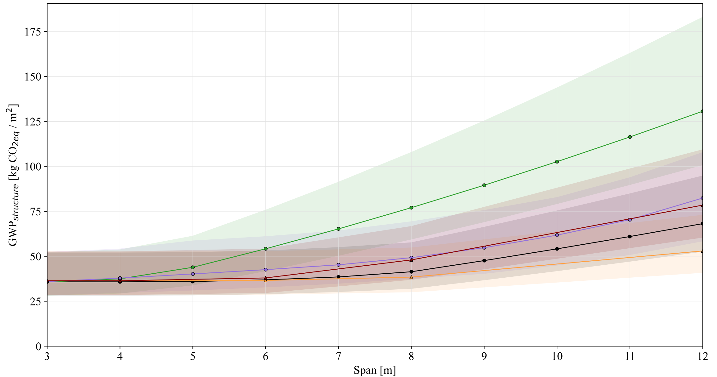
GWP Struktur inkl. Datenstreuung für 2D-Systeme & Referenz (Bodenaufbau Standard)
