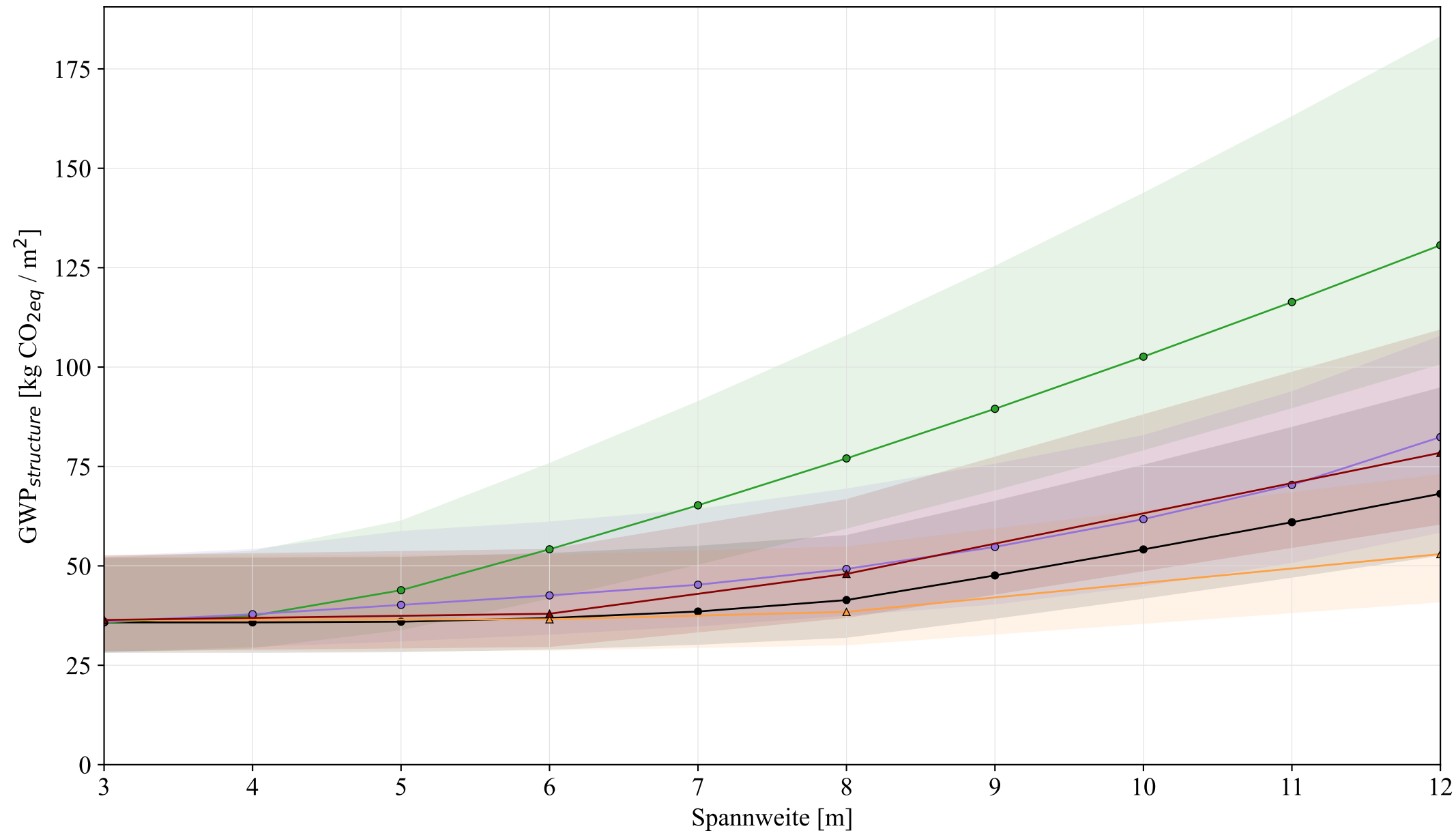
GWP Struktur inkl. Datenstreuung für 2D-Systeme & Referenz (Bodenaufbau Standard)
