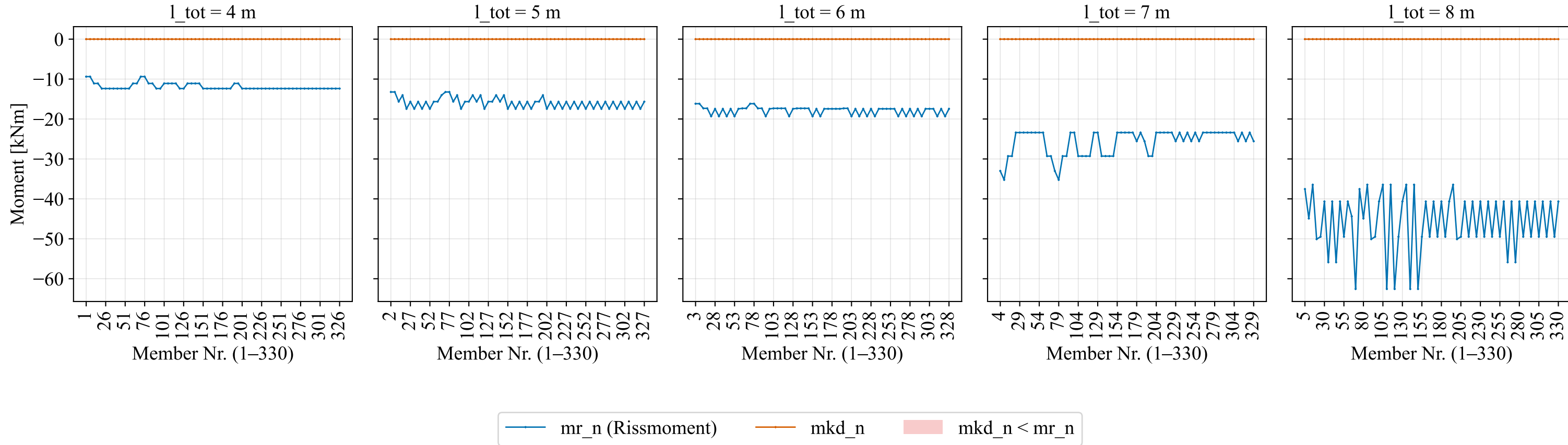
Rissmoment mr_n vs. Moment mkd_n (negative Biegung) je Member, kategorisiert nach Spannweite (Members_rc_rec_simple_massiv)
