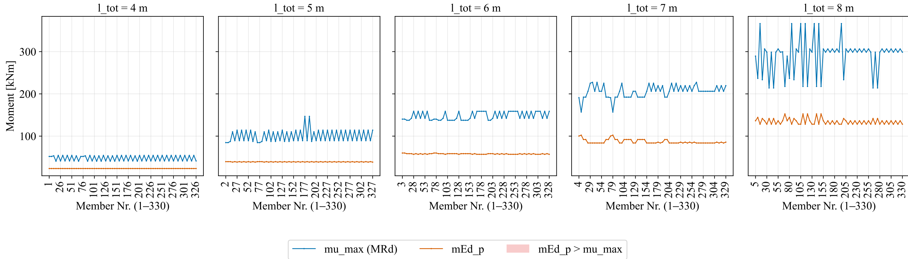
Biege widerstand \mu_{\max} (MRd) vs. Bemessungsmoment mEd_p je Member, kategorisiert nach Spannweite (Members_rc_rec_simple_massiv)
