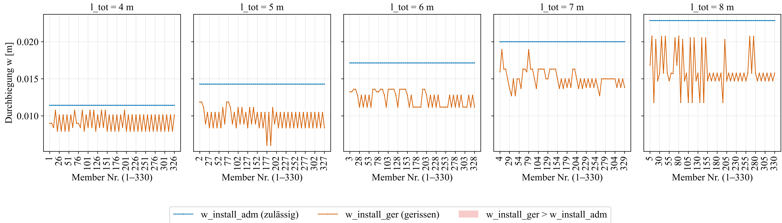
Durchbiegung w_{\text{install\_adm}} (zulässig) vs. w_{\text{install\_ger}} (Durchbiegung gerissen) je Member, kategorisiert nach Spannweite (Members_rc_rec_simple_massiv)
