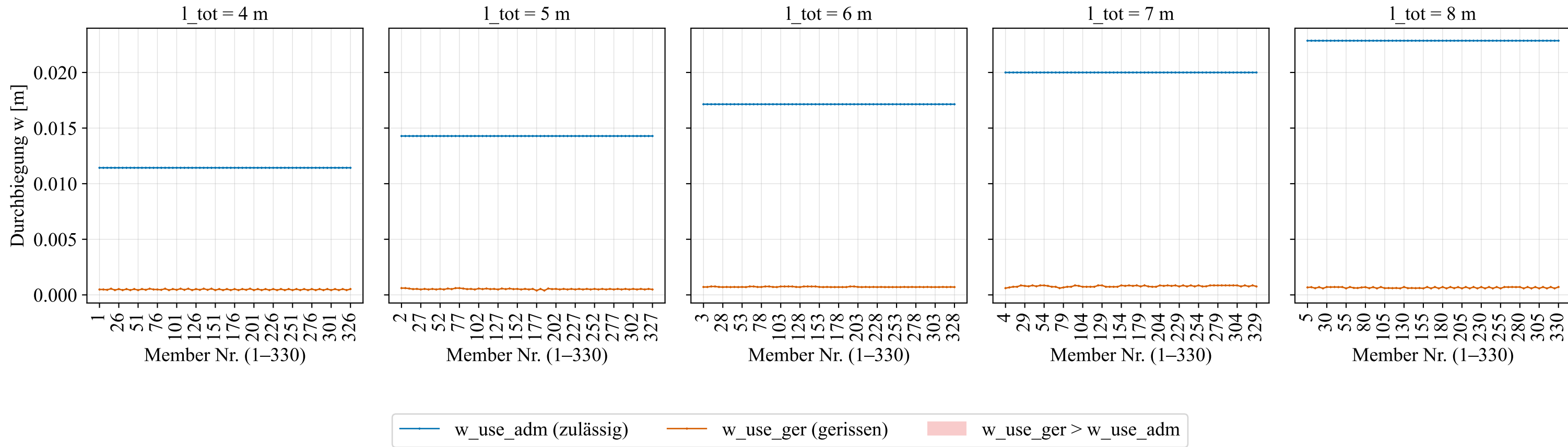
Durchbiegung w_{\text{use\_adm}} (zulässig) vs. w_{\text{use\_ger}} (gerissen) je Member, kategorisiert nach Spannweite (Members_rc_rec_simple_massiv)
