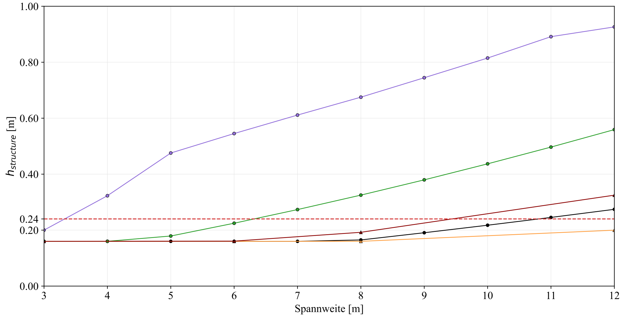
Höhe Struktur h_{struc} für Systeme mit Standardbodenaufbau
