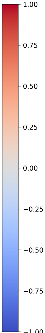
1.00 0.00 -0.00 0.00 0.00 0.00 0.00 -0.00 0.00 0.00 0.00 1.00 0.00 0.00 -0.00 -0.00 -0.00 0.00 -0.00 -0.00 -0.00 0.00 1.00 1.00 -0.00 -0.00 -0.00 0.00 0.00 0.00 0.00 0.00 1.00 1.00 0.00 0.00 0.01 -0.01 0.00 -0.00 0.00 -0.00 -0.00 0.00 1.00 1.00 0.00 0.03 0.00 -0.00 0.00 -0.00 -0.00 0.00 1.00 1.00 0.00 0.03 0.00 -0.00 0.00 -0.00 -0.00 0.01 0.00 0.00 1.00 -0.73 0.00 -0.00 -0.00 0.00 0.00 -0.01 0.03 0.03 -0.73 1.00 0.00 -0.00 0.00 -0.00 0.00 0.00 0.00 0.00 0.00 0.00 1.00 -0.00 0.00 -0.00 0.00 -0.00 -0.00 -0.00 -0.00 -0.00 -0.00 1.00
