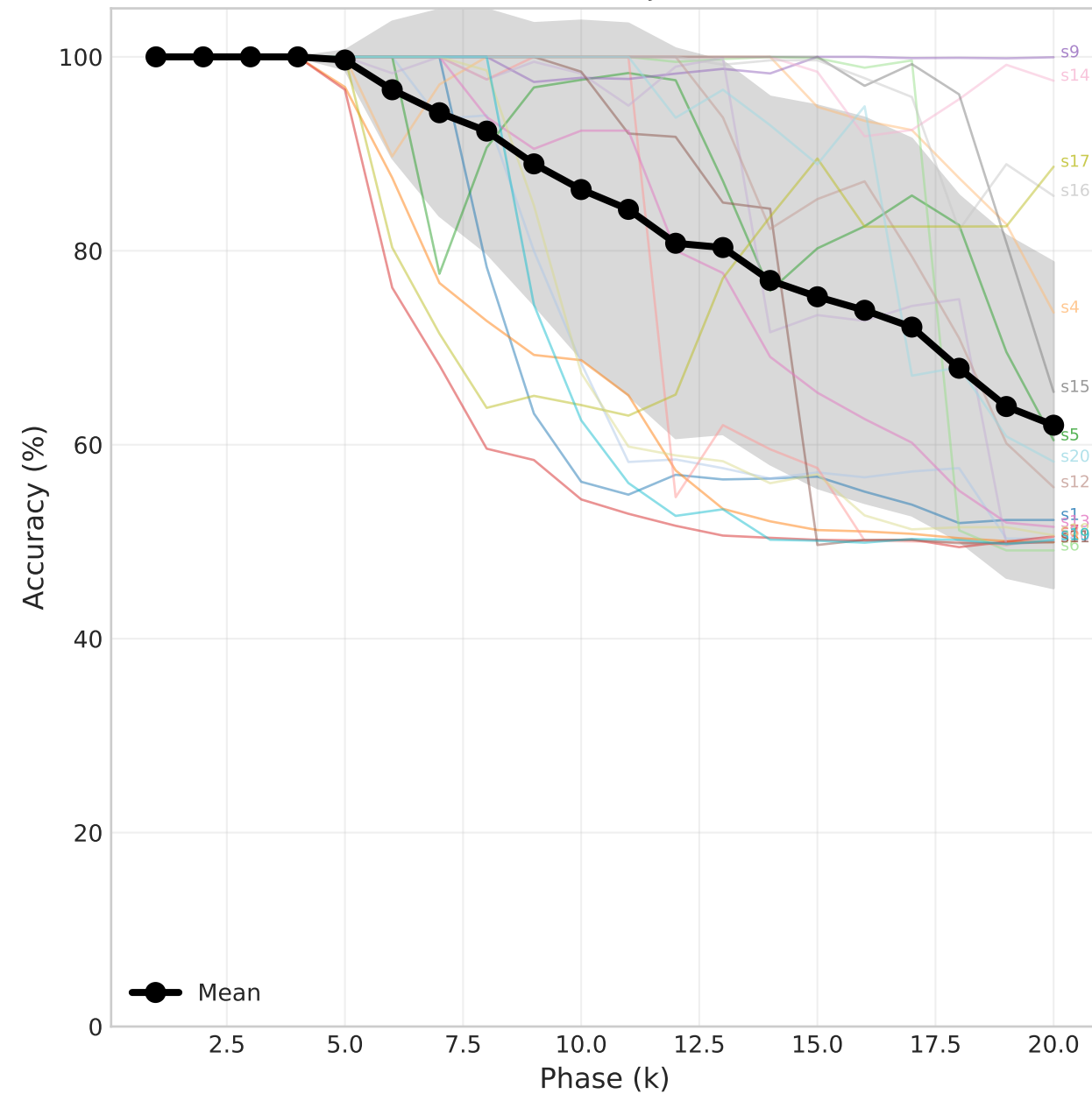
No CoT: All Trajectories
