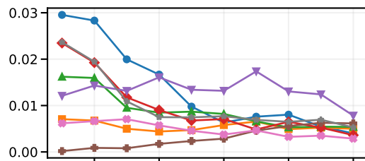
Macro-F1
