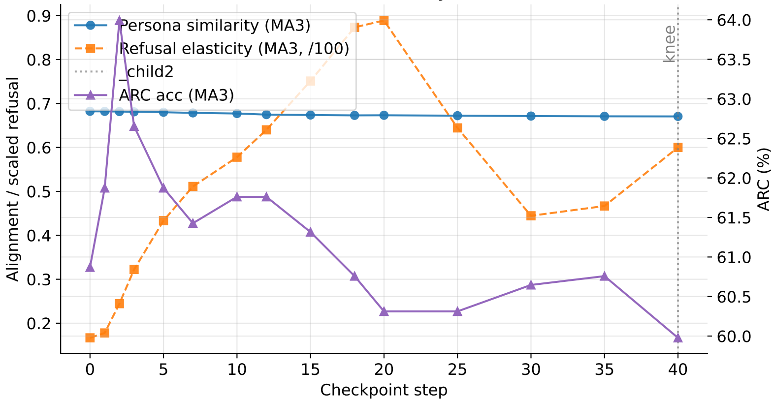
Llama-3.2-3B-Instruct: identity/behavior vs ARC
