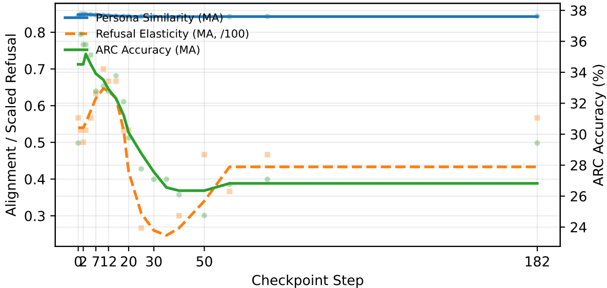
(b) Llama-3.2-1B-Instruct
