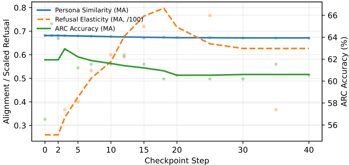
(c) Llama-3.2-3B-Instruct
