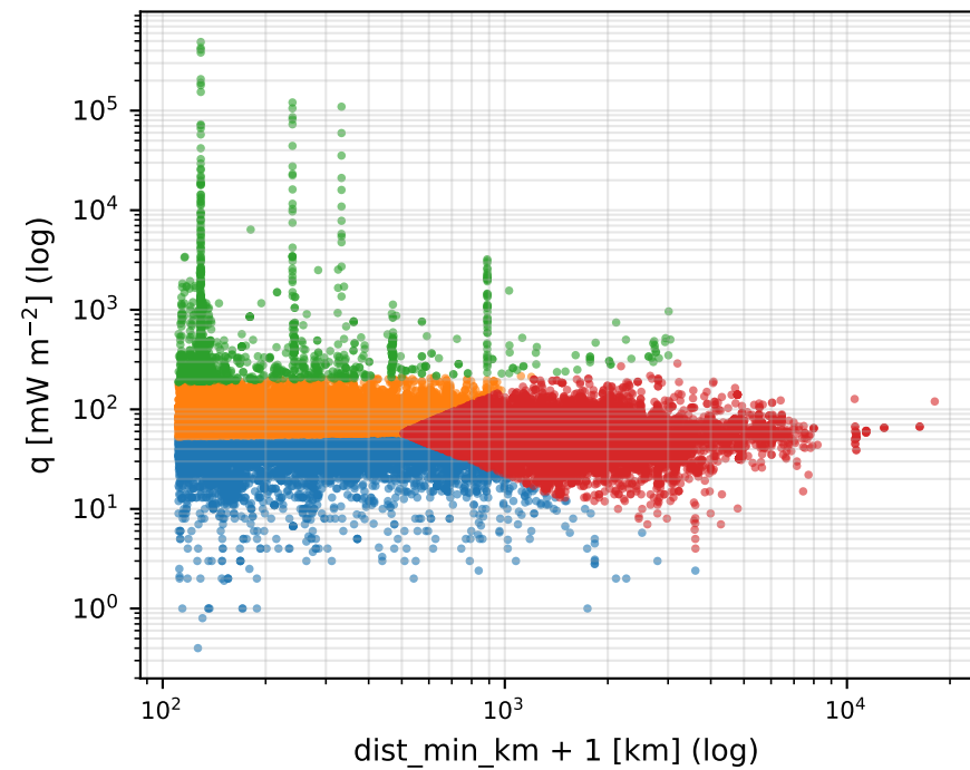
K-Means (k=4)
