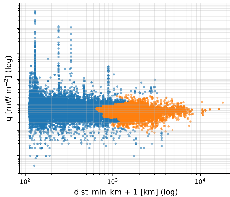
Hier/Ward (k=2)
