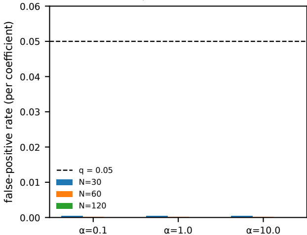
C4 null: per-coefficient FP rate
