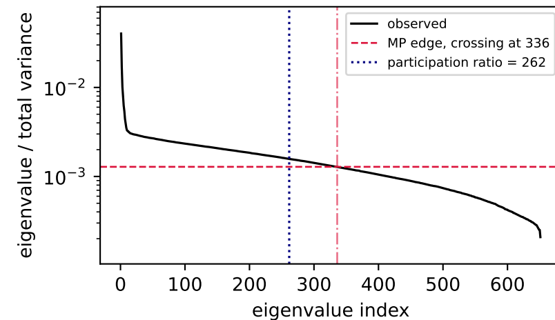
rpe1 n=8000, p=651 rank 651/651
